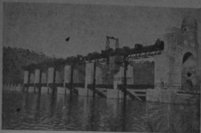
Parte baja de la genial prensa que contiene el empuje de muchos millones de litros de agua, que el hombre ha convertido en riqueza fecunda y gloriosa.
